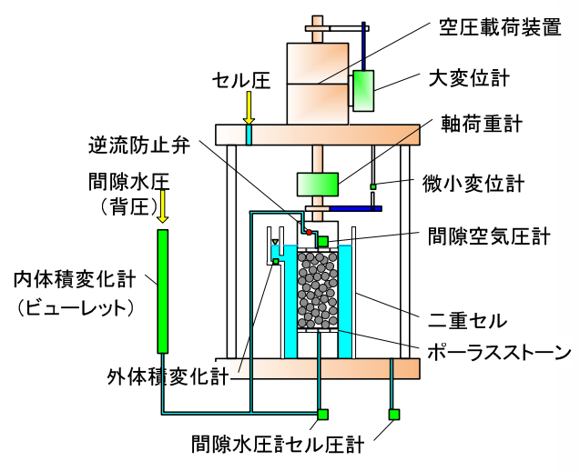
不飽和繰返し三軸試験装置概要
