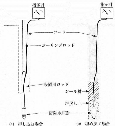
図-2 電気式間隙水圧計の設置例
