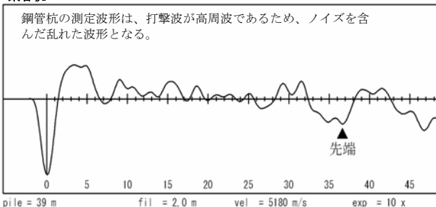
図-5 鋼管杭
