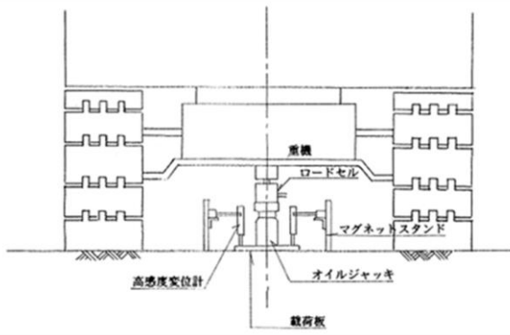
図-1 道路の平板載荷試験の測定概念図
