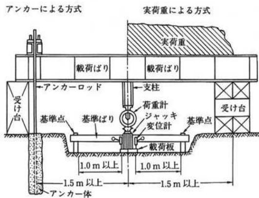
図-1 平板載荷試験の測定概念図
