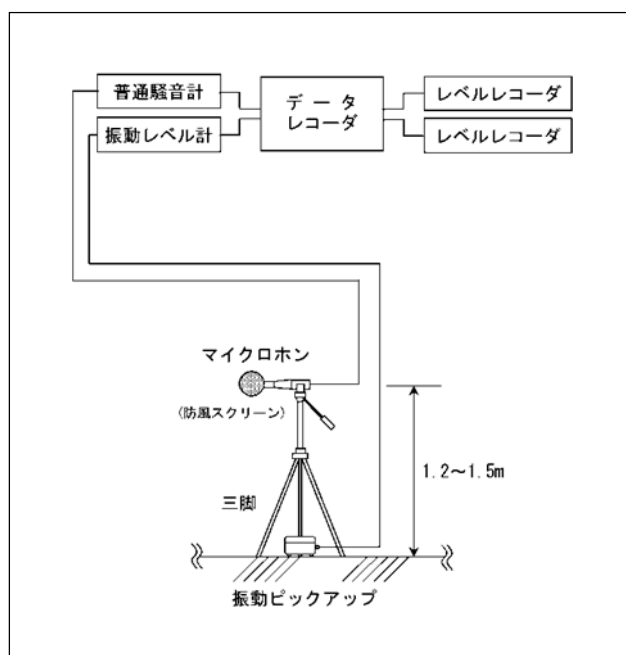
図-1 騒音・振動計測概念図
