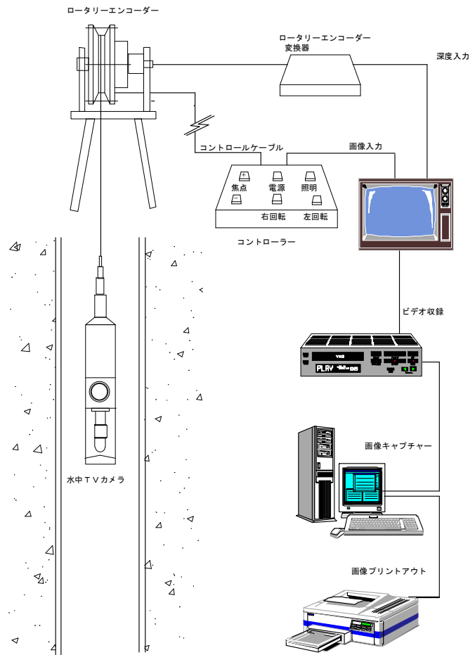
PIC 方式カメラシステム概念図
