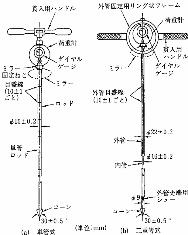
図-1 ポータブルコーン貫入試験機の例
